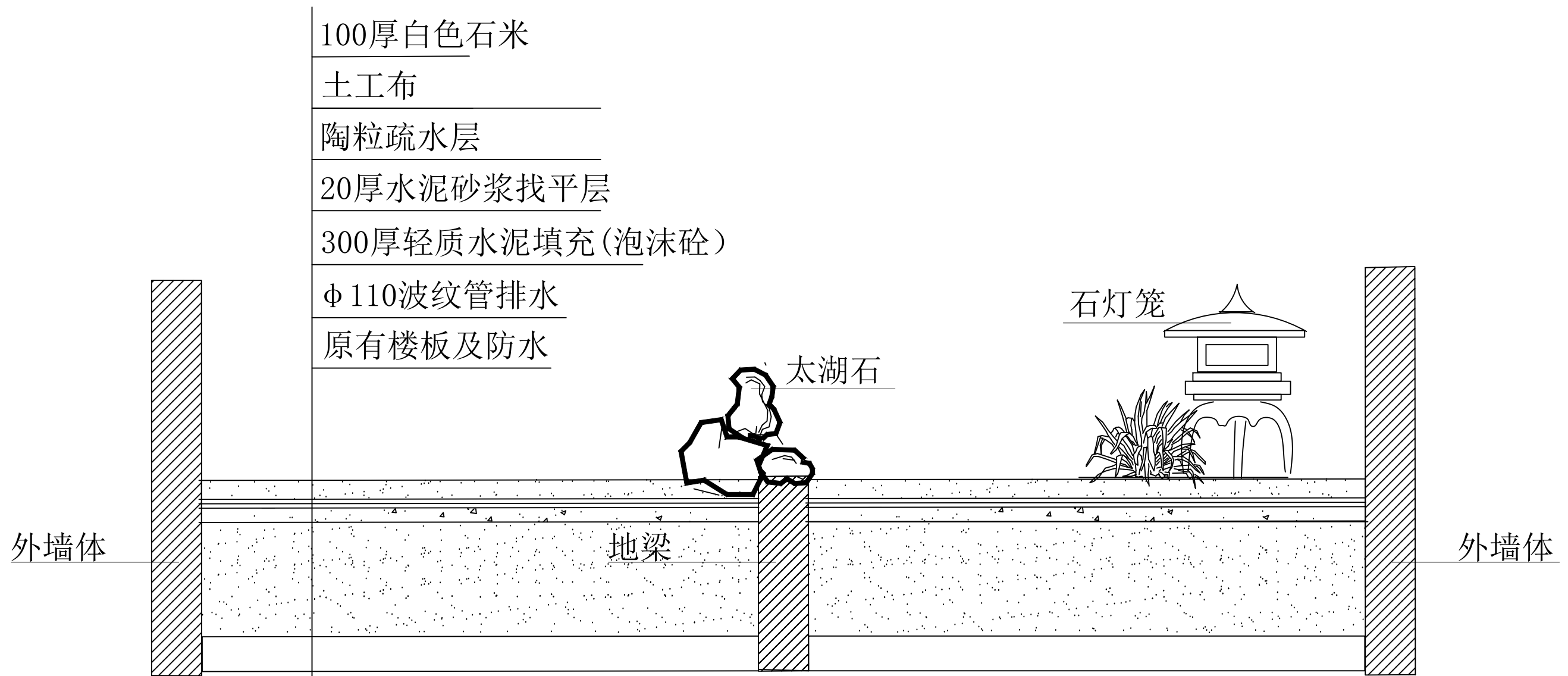
1-1枯山水结构剖面图1: 60
